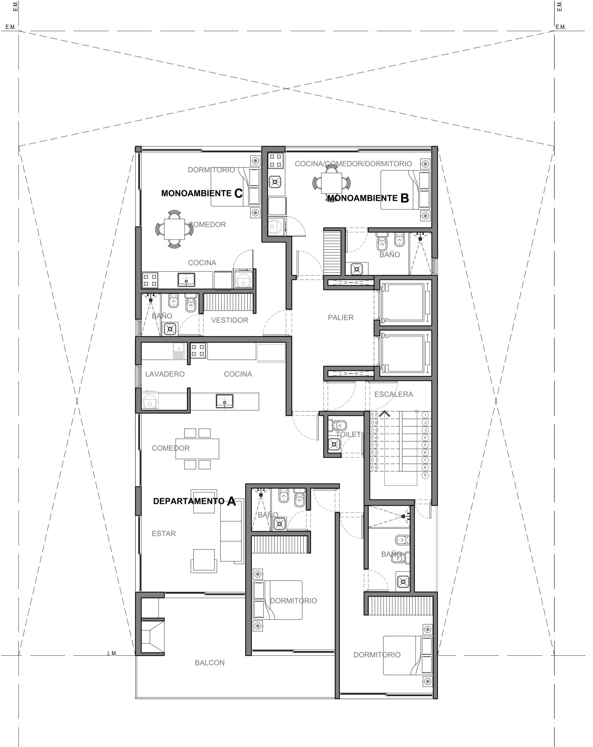
PLANTA 7° PISO
